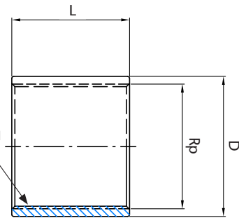
Taraudage cylindrique femelle Rp - EN 10226-1 et ISO 7-1 Female parallel thread Rp - EN 10226-1 and ISO 7-1
