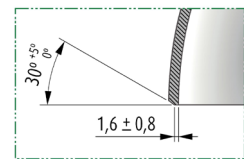
Chanfrein d'extrémité End chamfer
